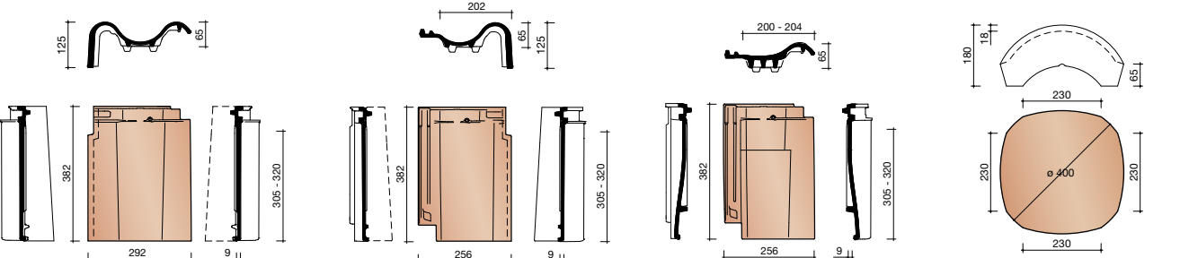
Vėjalentinė čerpė kairė Vėjalentinė čerpė dešinė Ventiliacinė čerpė X tipo čerpė
