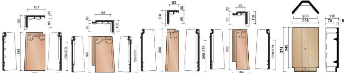
Vėjalentinė čerpė kairė Vėjalentinė čerpė dešinė 1/2 (pusinė) vėjalentinė čerpė kairė 1/2 (pusinė) vėjalentinė čerpė dešinė Kraigo čerpė
