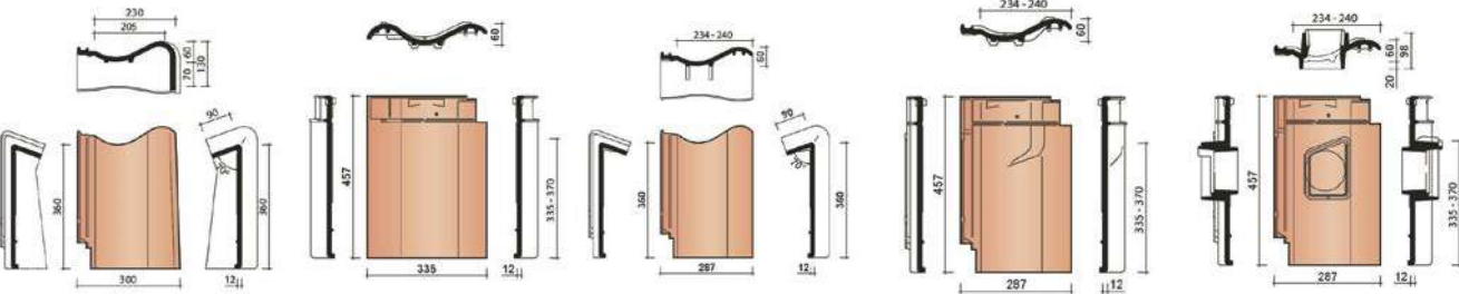
Vienšlaičio kraigo čerpė dešinė Dvibangė čerpė Vienšlaičio kraigo čerpė Ventiliacinė čerpė Ventiliacinis kaminėlis Ø100 mm
