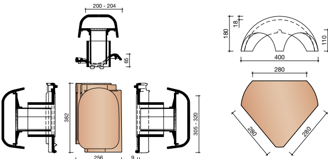
Keraminis ventiliacinis kaminėlis Ø 125 mm Y tipo čerpė
