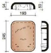
Ventiliacinio kaminėlio kepurėlė Ø100 mm
