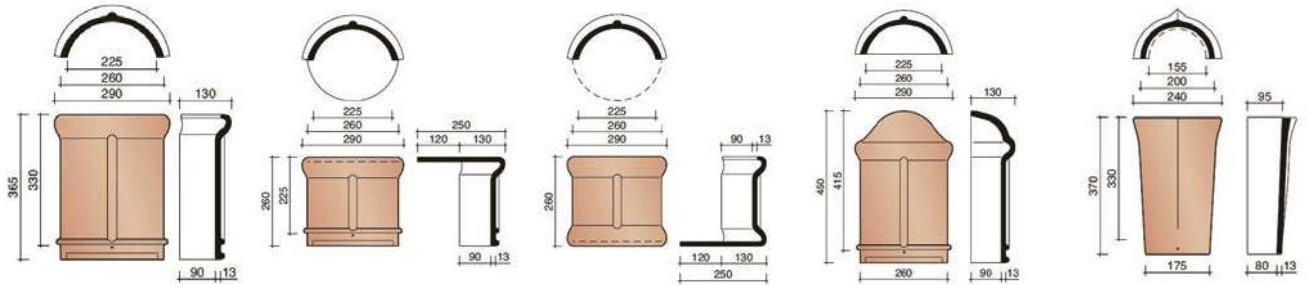
Kraigo čerpė Kraigo pradžia dangtelis Kraigo pabaigos dangtelis Valminio kraigo pradžia čerpė Valminio kraigo čerpė
