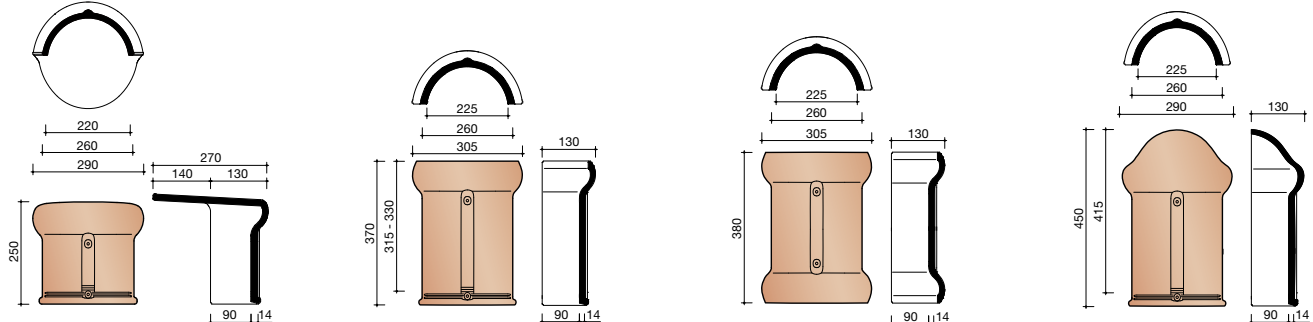
Kraigo pradžios/pabaigos dangtelis Kraigo čerpė Dvipusė kraigo čerpė Valminio kraigo pradžios čerpė
