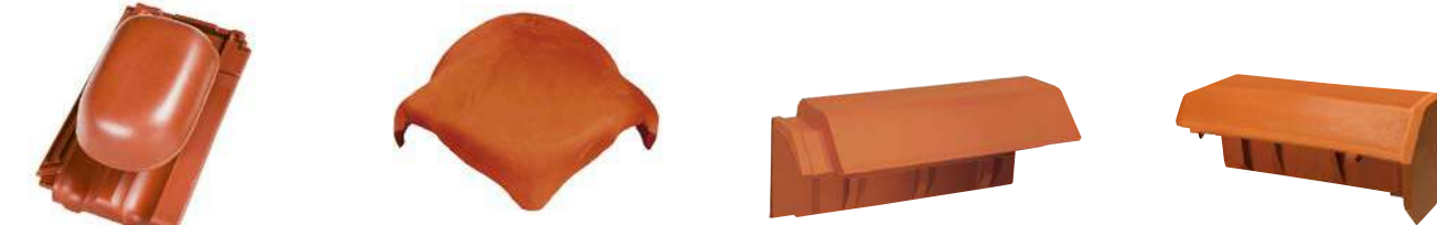
Ventiliacinis kaminėlis Valminė universali kraigo čerpė Nr. 1 (Y forma) Vienšlaičio kraigo čerpė Vienšlaičio kraigo pradžios čerpė
