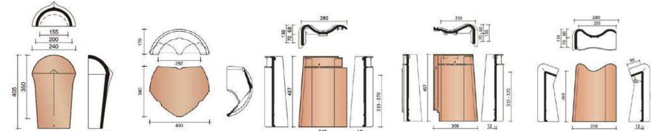
Valminio kraigo pradžia čerpė Valminė universalinė kraigo čerpė (Y-formos) Vėjalentinė čerpė kairė Vėjalentinė čerpė dešinė Vienšlaičio kraigo čerpė kairė
