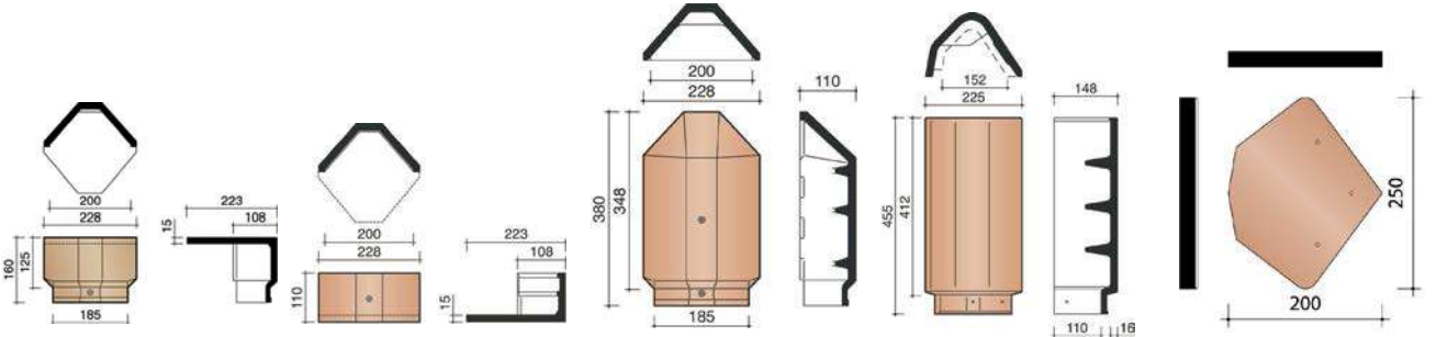
Kraigo pradžios dangtelis Kraigo pabaigos dangtelis Valminio kraigo pradžios čerpė Vienšlaičio kraigo čerpė Vienšlaičio kraigo pradžios/pabaigos dangtelis
