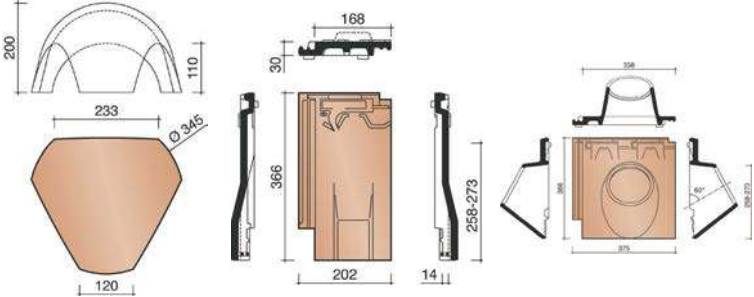
Valminė universali kraigo čerpė (Y-formos) Ventiliacinė čerpė Ventiliacinis kaminėlis Ø150 mm
